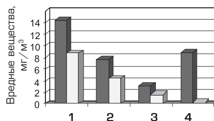
Рис. 28. Эмиссия вредных веществ на участке выбивки: 1 – бензол; 2 – толуол; 3 – ксилол; 4 – фенол. Темные столбцы – немодифицированная система; светлые столбцы – модифицированная система
