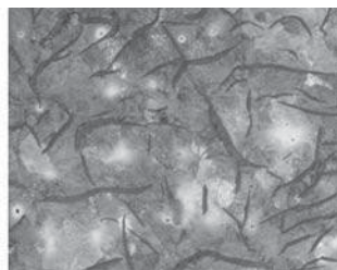
Рис. 12. Отливки №3, 4. Металлическая основа – перлит пластинчатый, следы феррита (травление – нитал) (x400)
